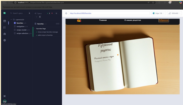
Cypress тестирование работы избранного
